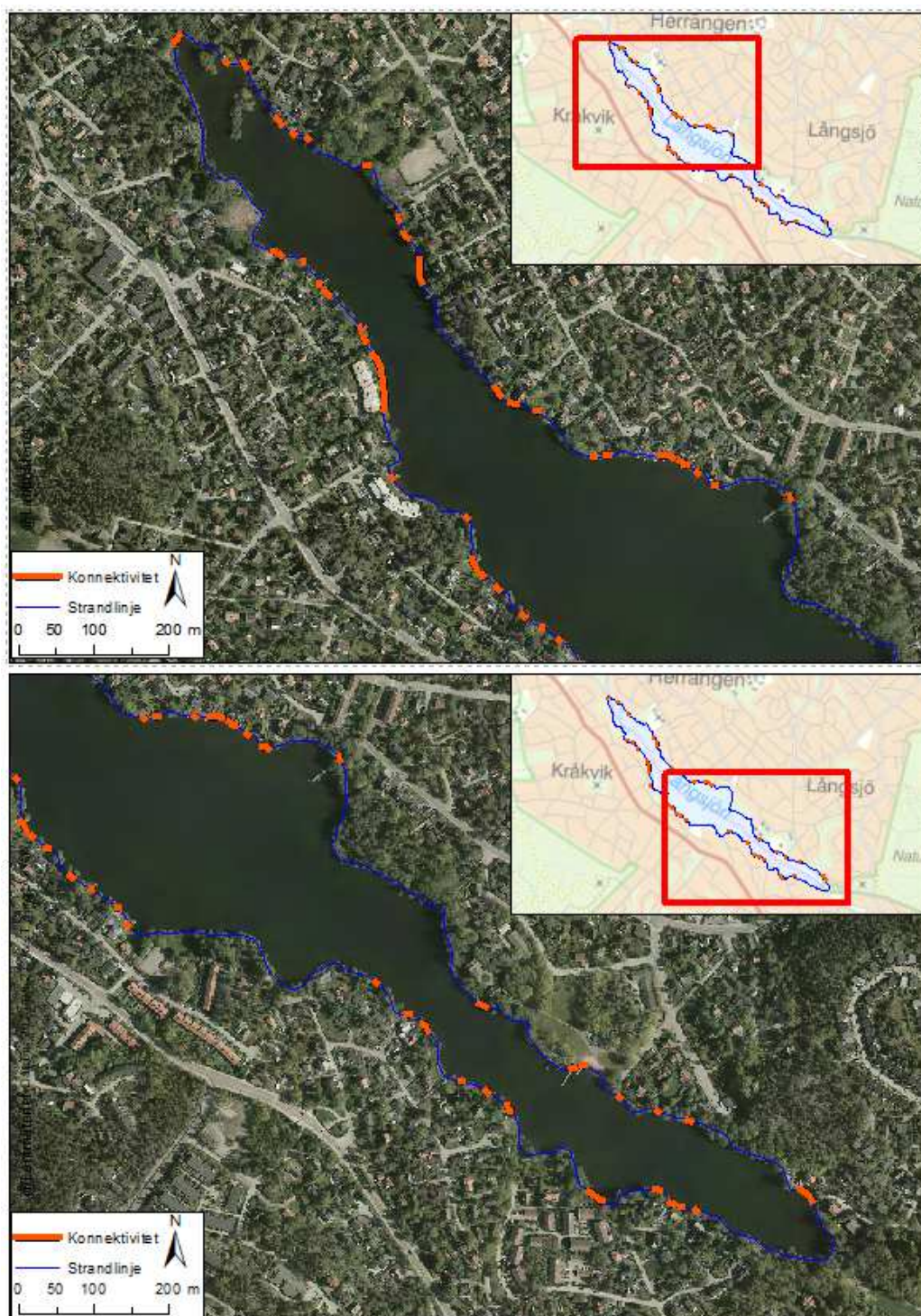
Figur 10. Bedömning av konnektivitet till närområde och svämplan i Långsjön. De röda sträcken visar områdena som bedöms ha bristande konnektivitet.
