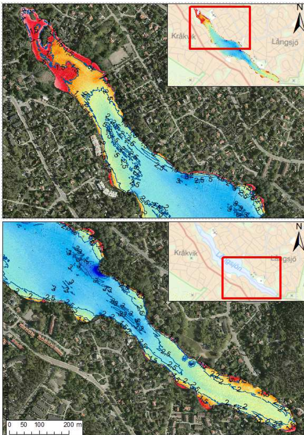
Figur 2. Översiktlig bild med djupkurvor i Långsjön. Färgerna visar djupgradients som komplement till djupkurvorna, rött 0-1,5 m, orange 1,5-2 m, grönt 2-2,5 m, ljusblått 2,5-3 m, mörkblått >3 m djup.
