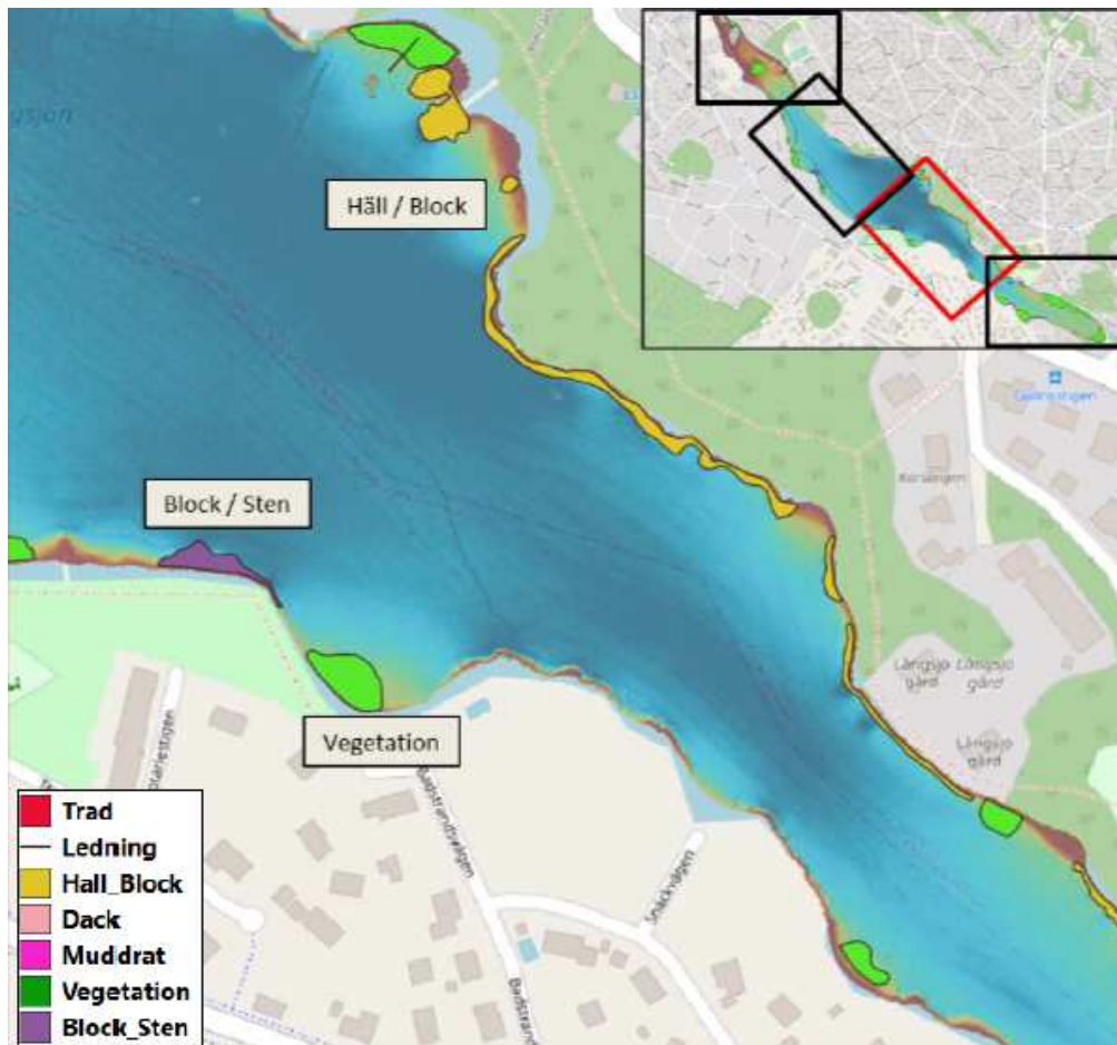
Figur 5. Tolkade strukturer från sjömätning av Långsjön, utförd av Clinton 2020. I den södra mellersta delen påträffades, ledning, muddrat område, block, häll och sten.
